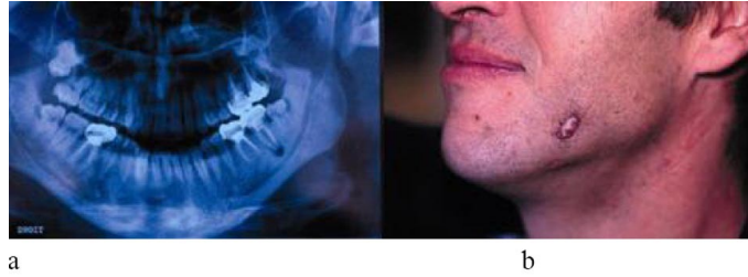
Figure 9.4 Granulome apical à l'origine de la fistule cutanée
