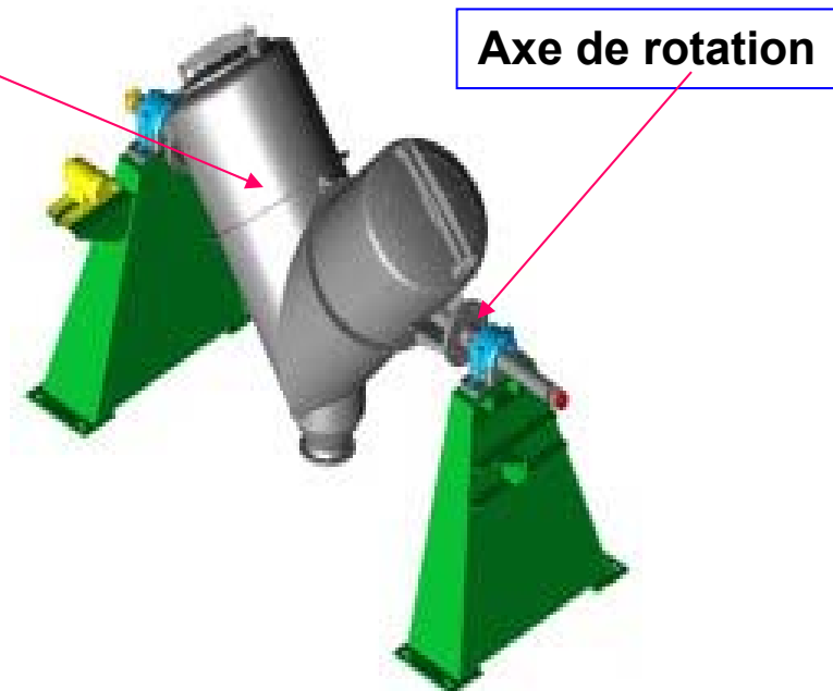
Mélangeur à tambour en V
