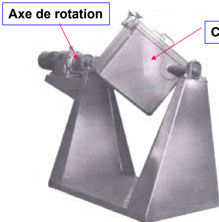
Mélangeur à tambour cubique
